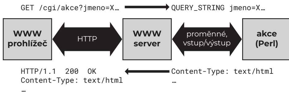
Obrázek 16.1: Rozhraní CGI
