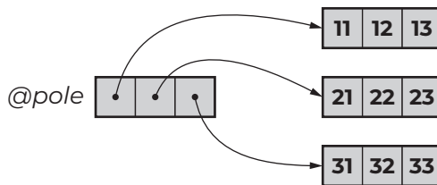
Obrázek 11.4: Dvojrozměrné pole
