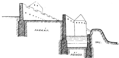
Průřez středověkým městským opevněním
