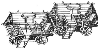
Sestavování vozové hradby způsobem "kolo na kolo" (vozy byly spojeny řetězy)
